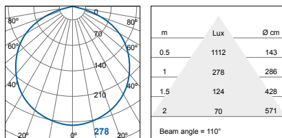
FIB76100v0-ps (3000K)
