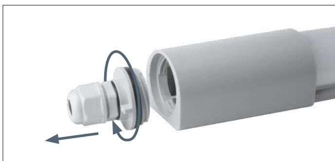
Tool-less wiring
