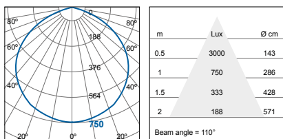
FFL71900v0-ps
